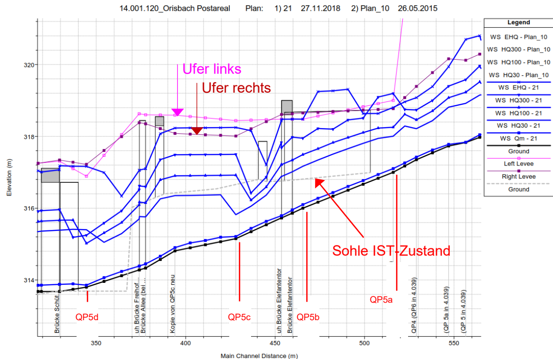
Abbildung 4 Längenprofil mit Wasserspiegel inkl. Vergleich Sohle IST-Zustand
